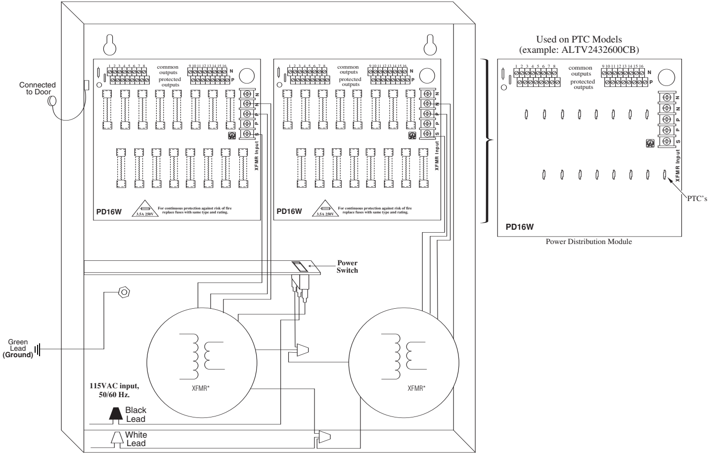
Fig. 3 ALTV2432600 • ALTV2432600CB
